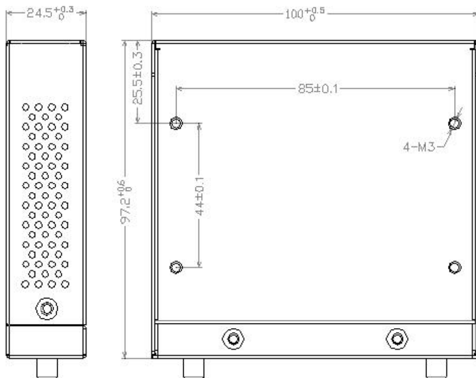
路由器尺寸
