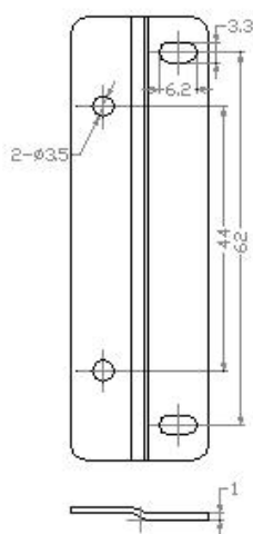
固定片尺寸
