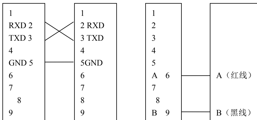
接口: RS232
